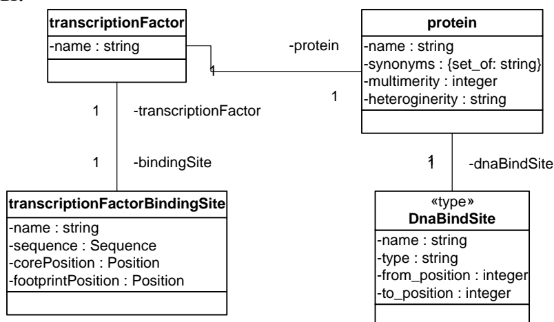
Рис.1 Фрагмент UML спецификации посредника
