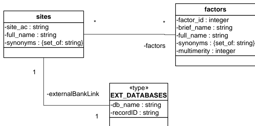
Рис.2 Фрагмент UML спецификации базы TRRD
