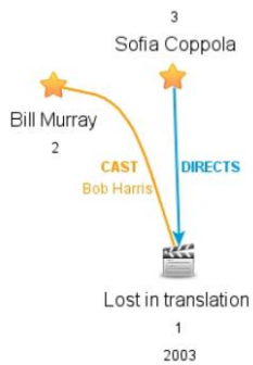
Рисунок 2. Пример графа в модели данных Neo4j
