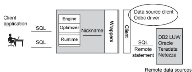
Рисунок 2. Архитектура BigSQL Federalization
