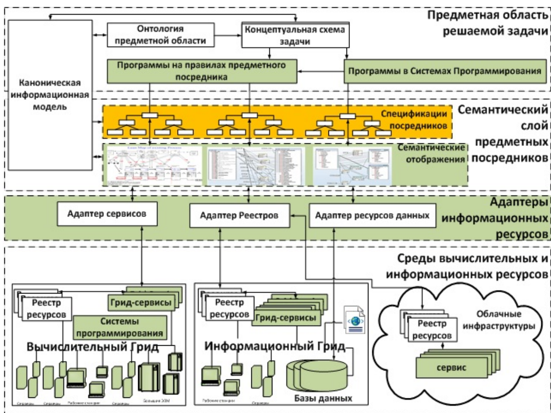
Рис. 1. Обобщенная архитектура среды предметных посредников
